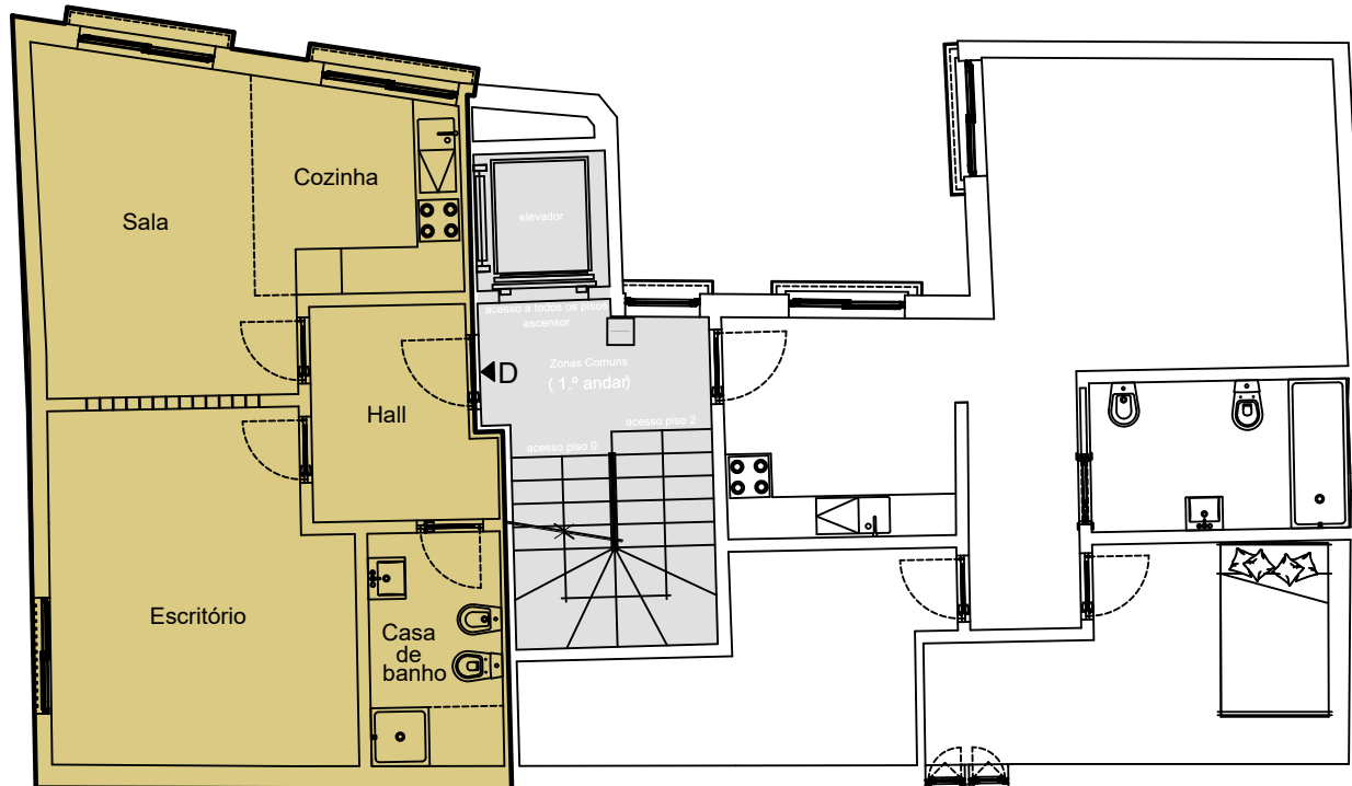
Escala 1:100 - Planta do Piso
